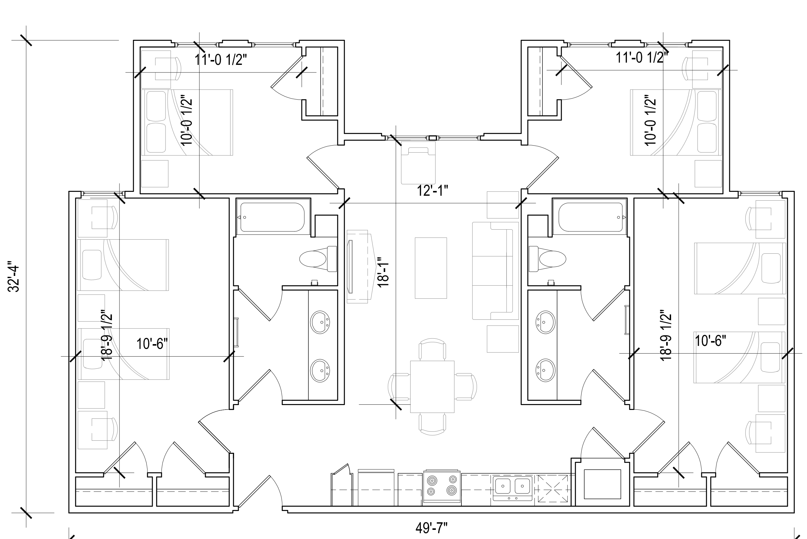
D-1 (1435 s.f.)
