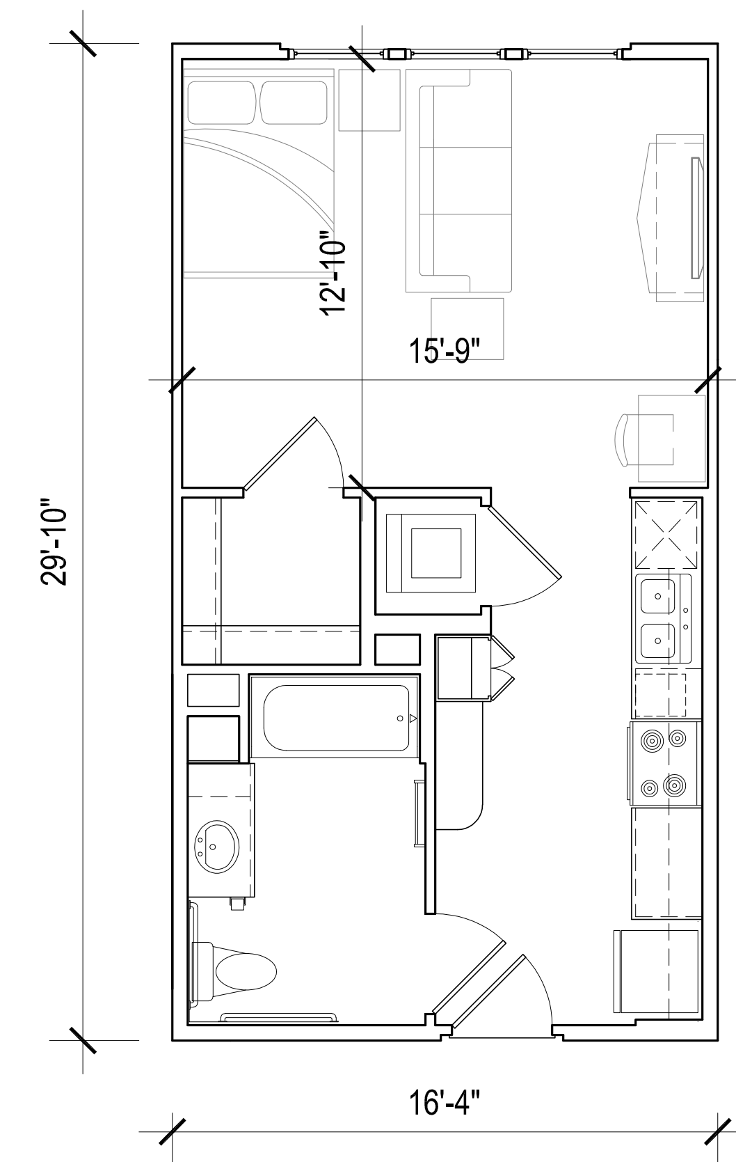
S-1 (487 s.f.)
